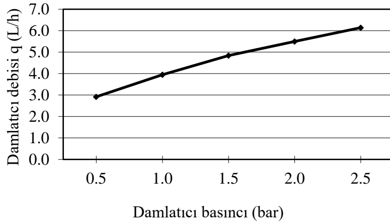
Şekil 2. SERTSAN damla sulama boruları (4.0 L/h anma debili, 16 mm anma çaplı)'nın damlatıcılarına ait basınç-debi ilişkisi
