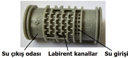
Şekil 1. SERTSAN damla sulama borularında (4.0 L/h anma debili) kullanılan silindirik damlatıcının genel görünüşü
