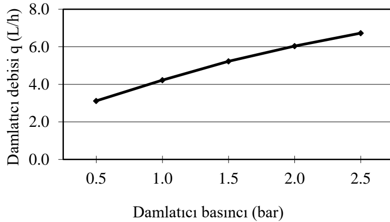
Şekil 2. SERTSAN damla sulama boruları (4.0 L/h anma debili, 20 mm anma çaplı)'nın damlatıcılarına ait basınç-debi ilişkisi
